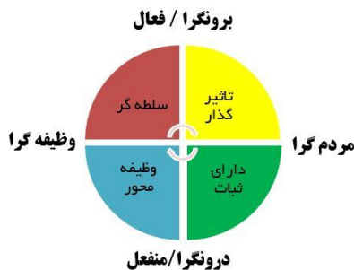
شکل ۴: مدل DISC
